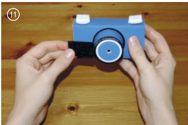
11. Сделать прорезь для затвора во внешнем объективе так, чтобы он мог попадать в механизм затвора на внутреннем объективе. Сделать аккуратно иголкой в фольге дырочку диаметром 0.4 мм.
